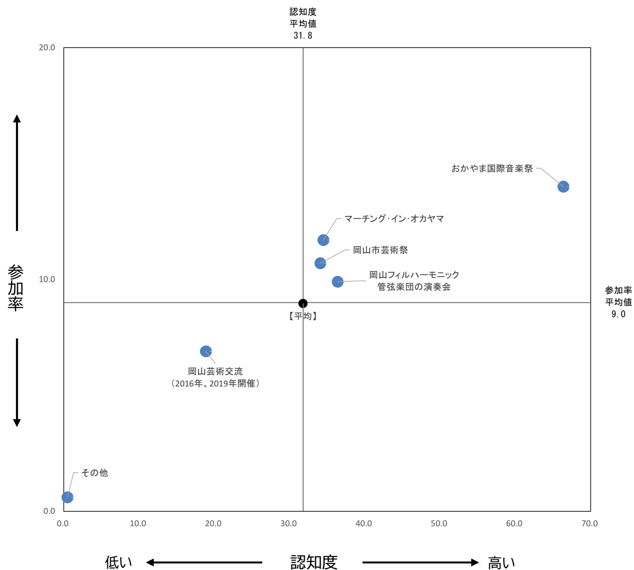
【散布図】
