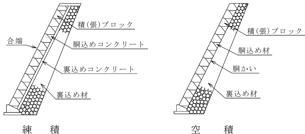
図2-5 コンクリートブロック工
