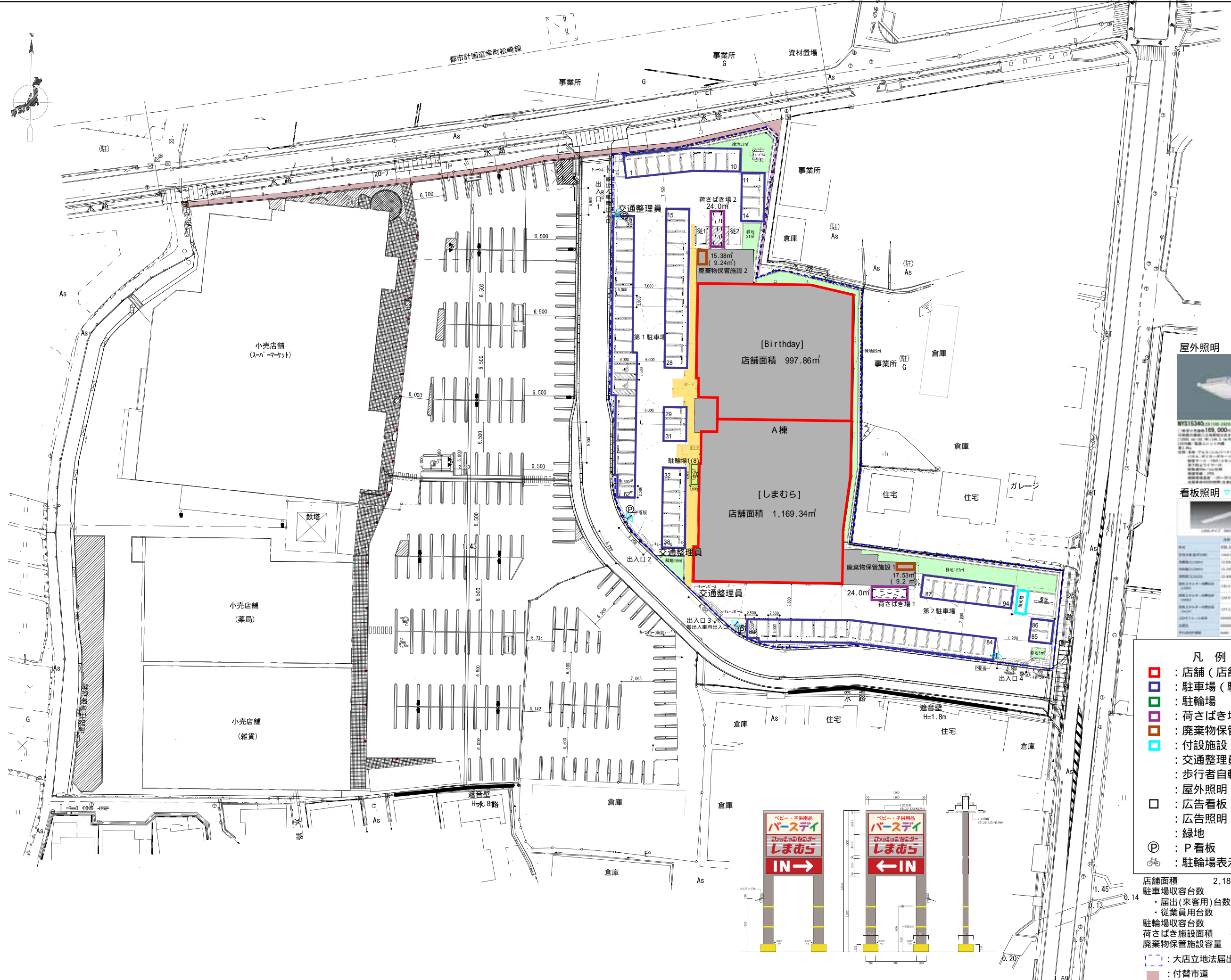
添付図3 配置図
