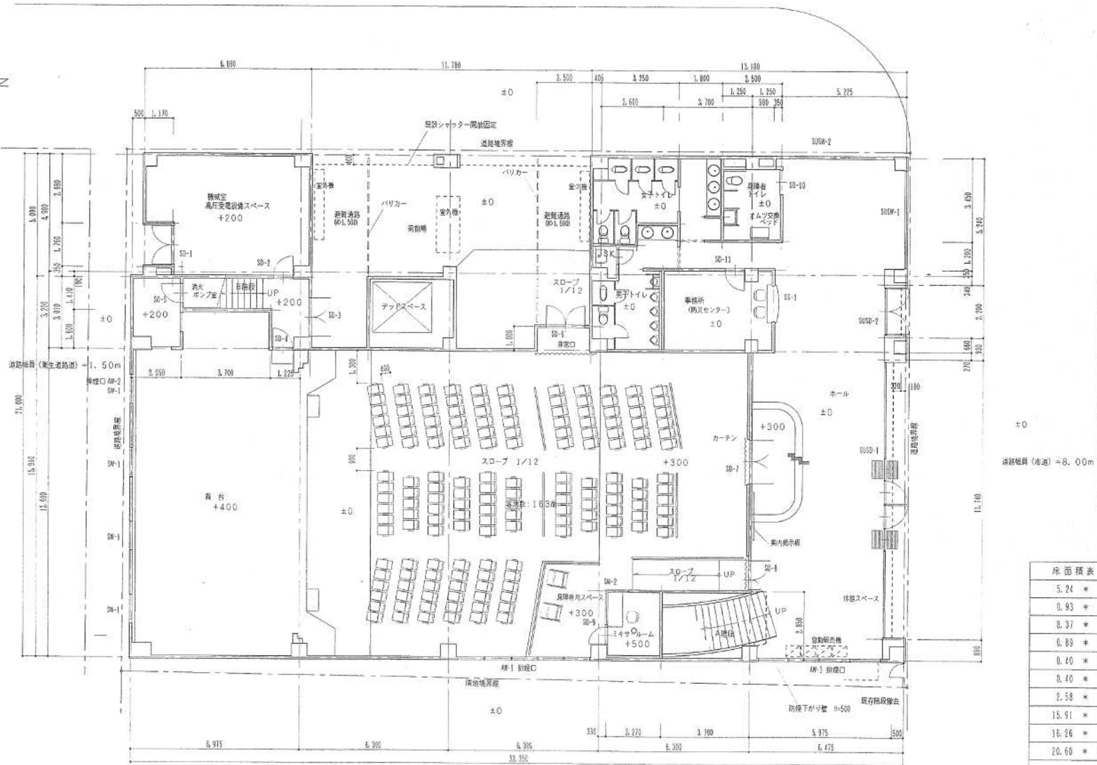
三丁目劇場 1階平面図
