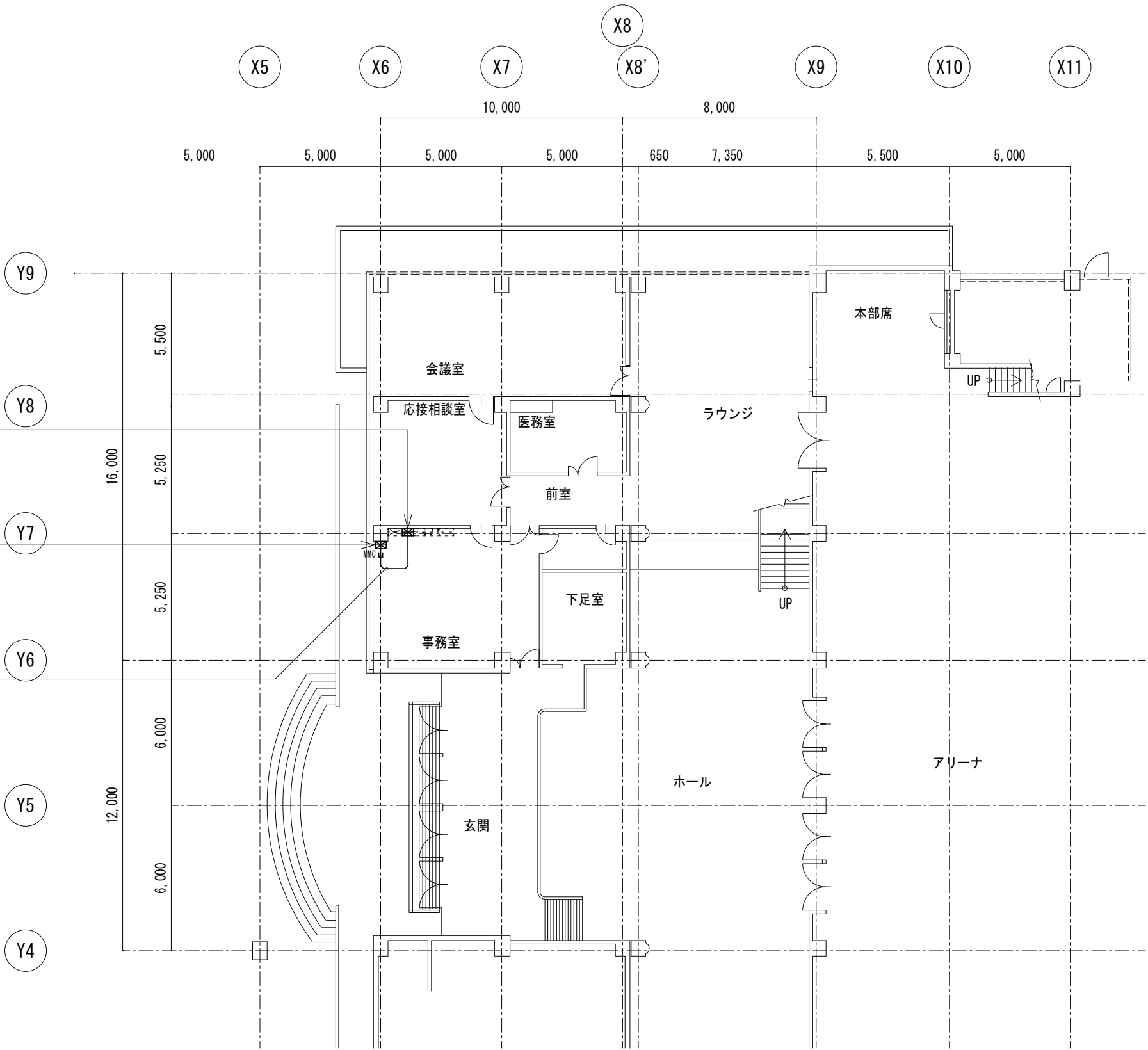
体育館（1階）平面図 【S=1:200】
