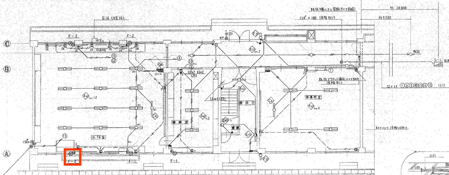
1階電灯コンセント設備平面図 S=1/100
