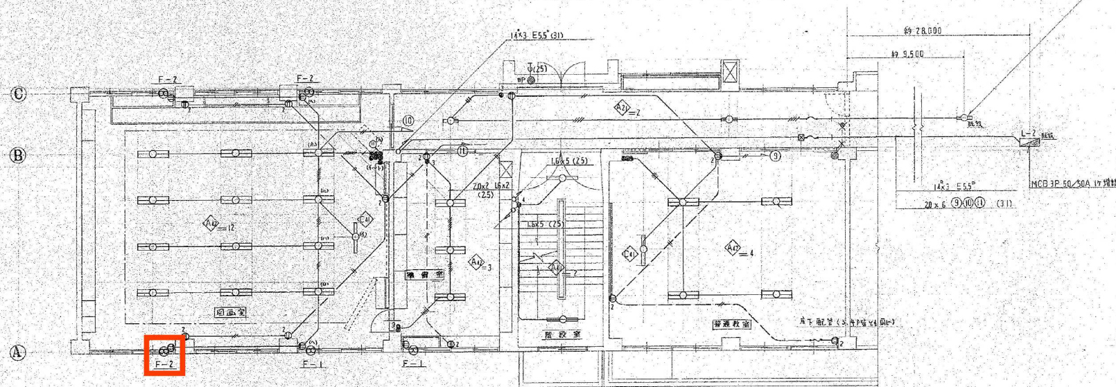
2階電灯コンセント設備平面図 S=1/100
