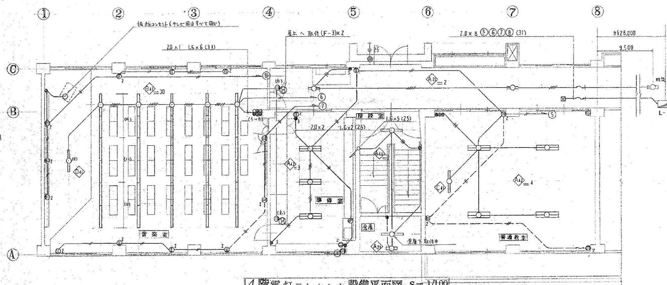
4階電灯コンセント設備平面図 S=1/100
