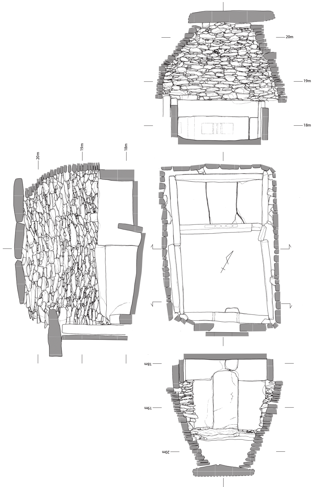
図5 千足古墳石室実測図 (1/50)
