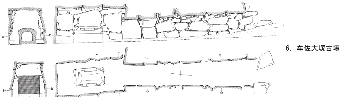
図4 吉備南部における横穴式石室の変遷 (1/2000)
