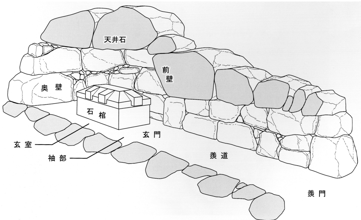
図1 「畿内型」石室の構造と部分名称
