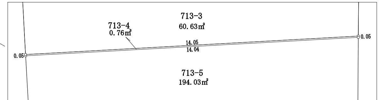
拡大図 (縮尺: 1/100)
