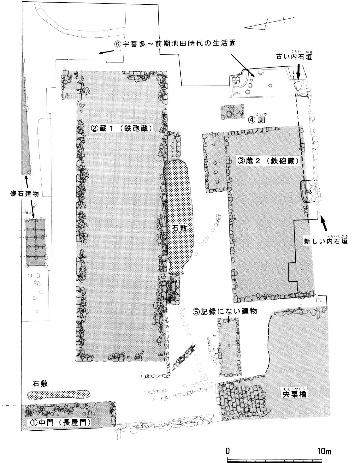
図 2 全体図 (S=1/200)
