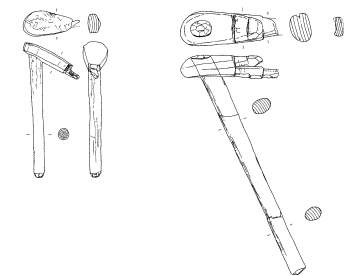
図5 一木と組合せの斧柄 南方（済生会）遺跡 (S=1/12)
