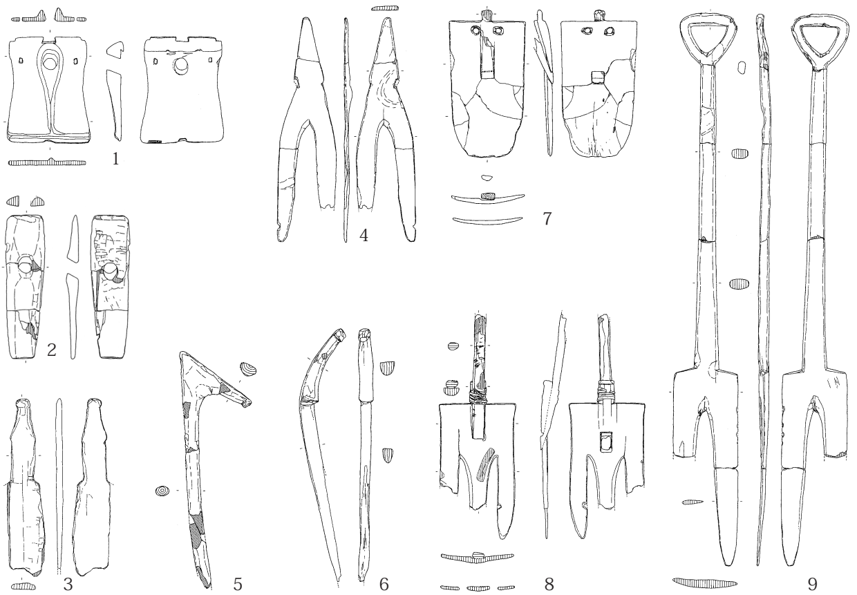
図3 南方（済生会）遺跡の鍬と鋤 (S=1/12)
