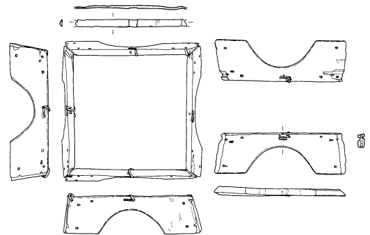
図9 青谷上寺地遺跡の指物 (S=1/8)
