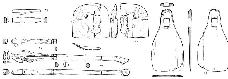
図4 北部九州の鍬の組合せ (S=1/12)
