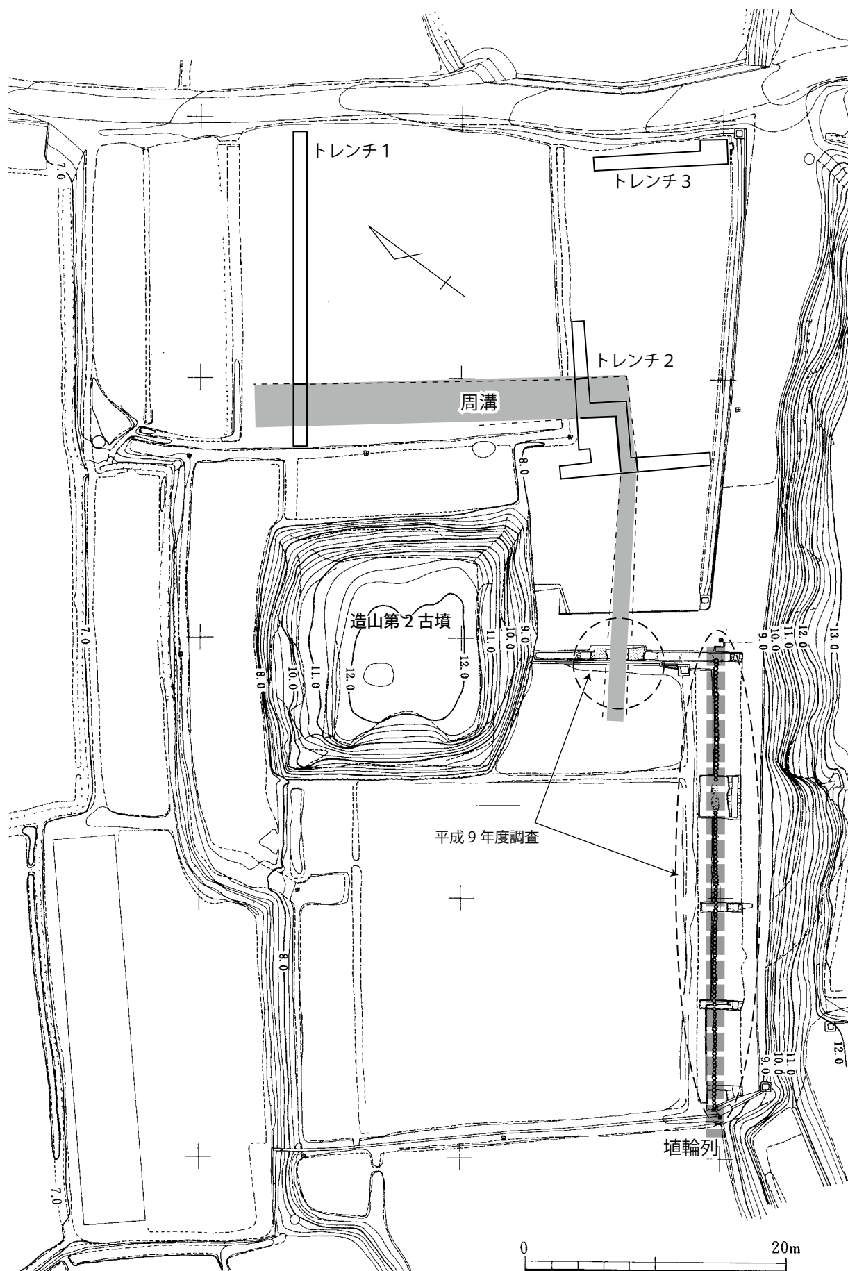
図2 造山第2古墳全体図 (1/400)
