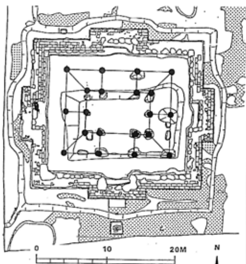
4、金堂建物遺構
