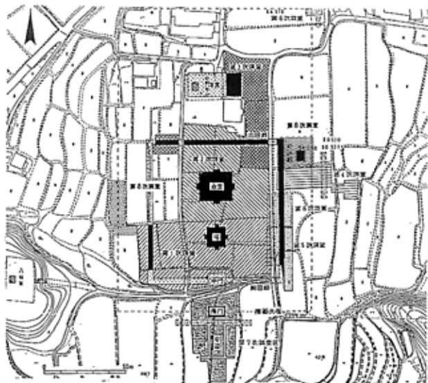
1、山田寺の地形と伽藍
