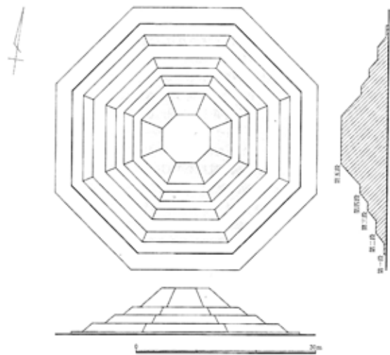
3、天武・持統天皇合葬陵復原図
