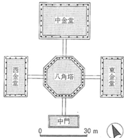
3、高句麗清岩里廃寺の伽藍
