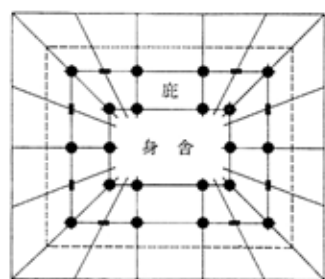
3、山田寺金堂の発掘
