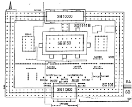
9 平城宮後期大極殿前庭の宝幢跡
