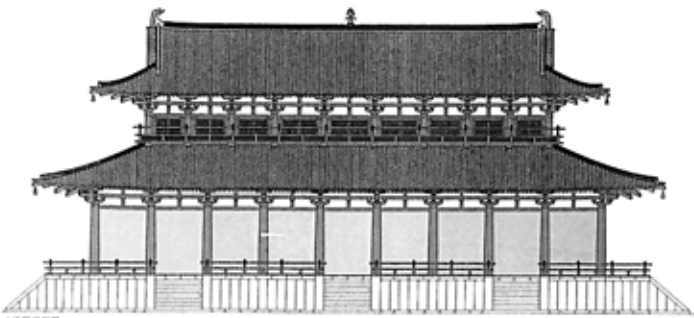
2、大極殿復原図
