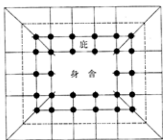
6、玉虫厨子建物と法隆寺金堂の礎石と垂木配置
