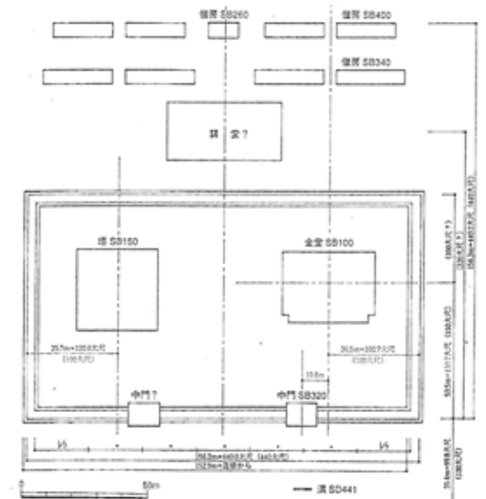
10、百濟大寺の伽藍復原図
