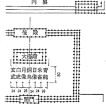
9 平城宮後期大極殿前庭の宝幢跡
