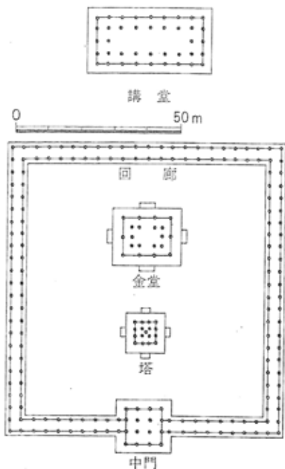
2、山田寺の伽藍配置
