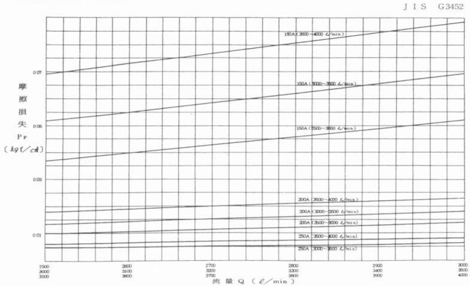
図3-9 等価管長1m当りの摩擦損失
