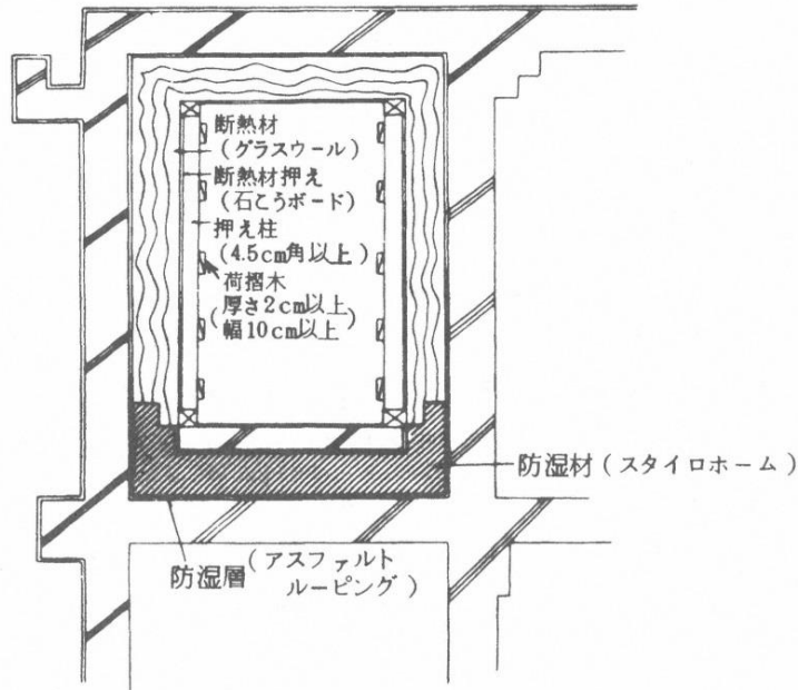
図6-2 冷凍室等断熱処理施工例
