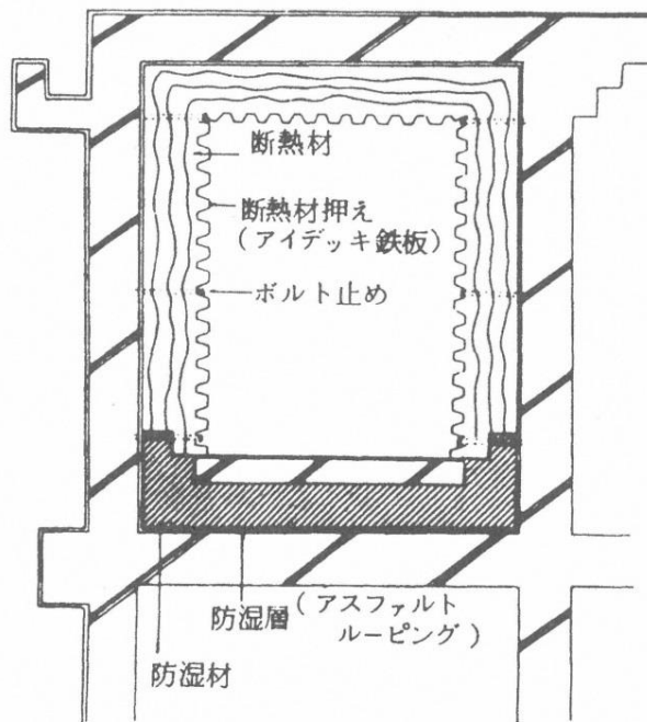
図6-2 冷凍室等断熱処理施工例
