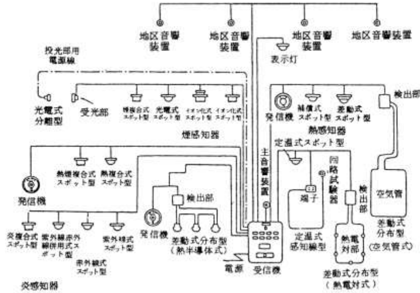
図10—1 自動火災報知設備の構成図例
