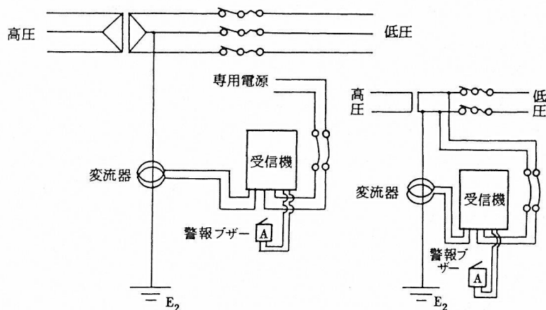
例 2 変圧器のB種接地線に設ける場合
