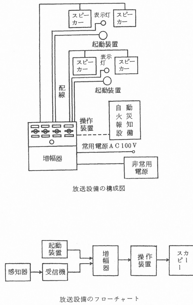
図14-4 非常放送設備の概要
