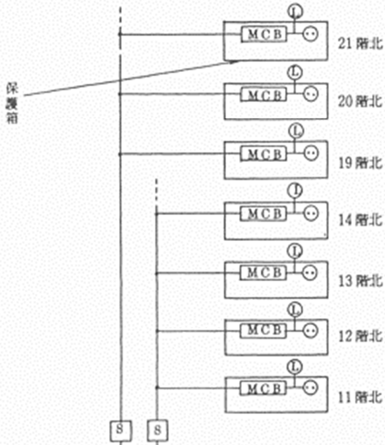
図21-1 非常コンセント設備の構成図例
