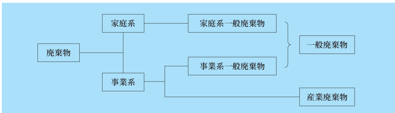
図37 廃棄物とは
