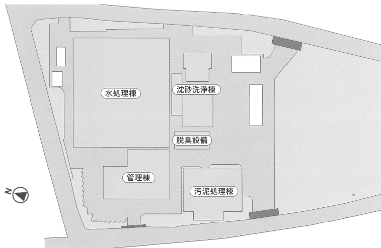
施設配置図
