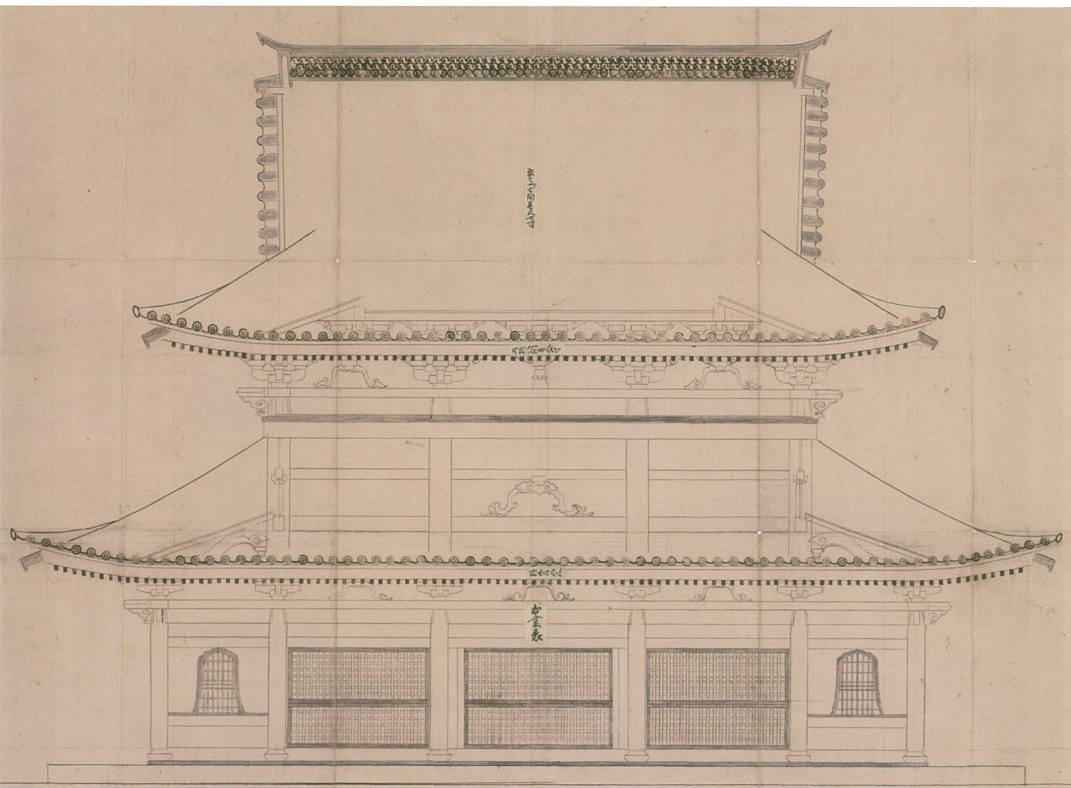
八塔寺本堂指図
