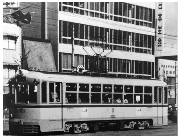
◎ 1000 形車両。車軸を多くし、可動式の台車を介することで車体を長くしたボギー車で、現在まで使用されている。(岡山電気軌道株式会社所蔵写真)
