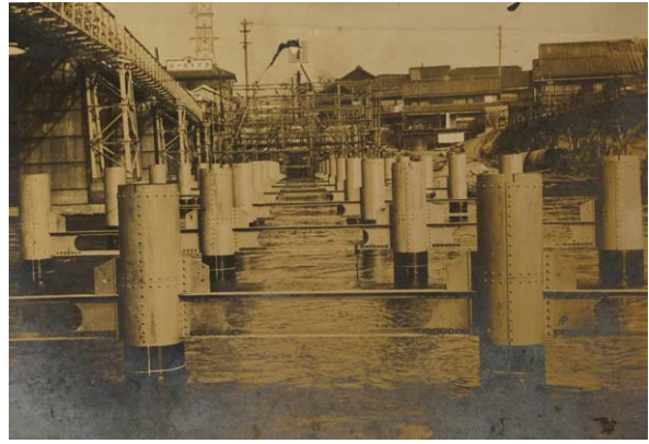
橋脚下部の鉄管の組み立て
