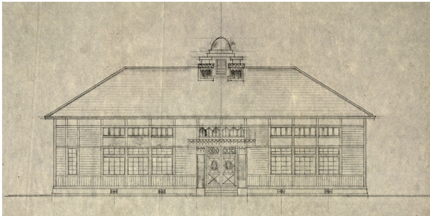
藤田尋常小学校講堂の設計図から(昭和4年)岡山市立中央図書館蔵
