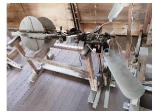
足踏み式製縄機
