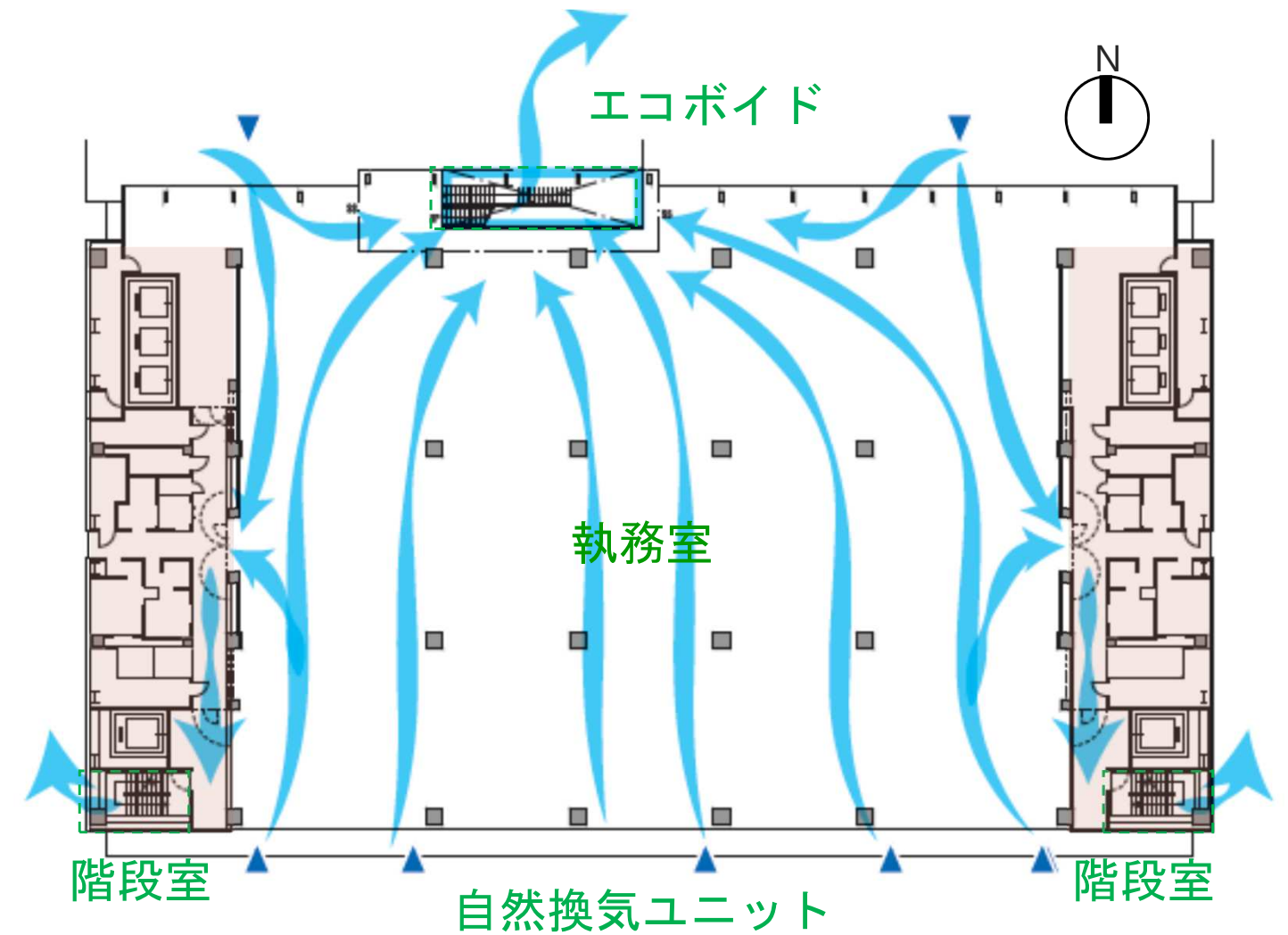
執務室フロアの自然換気イメージ
