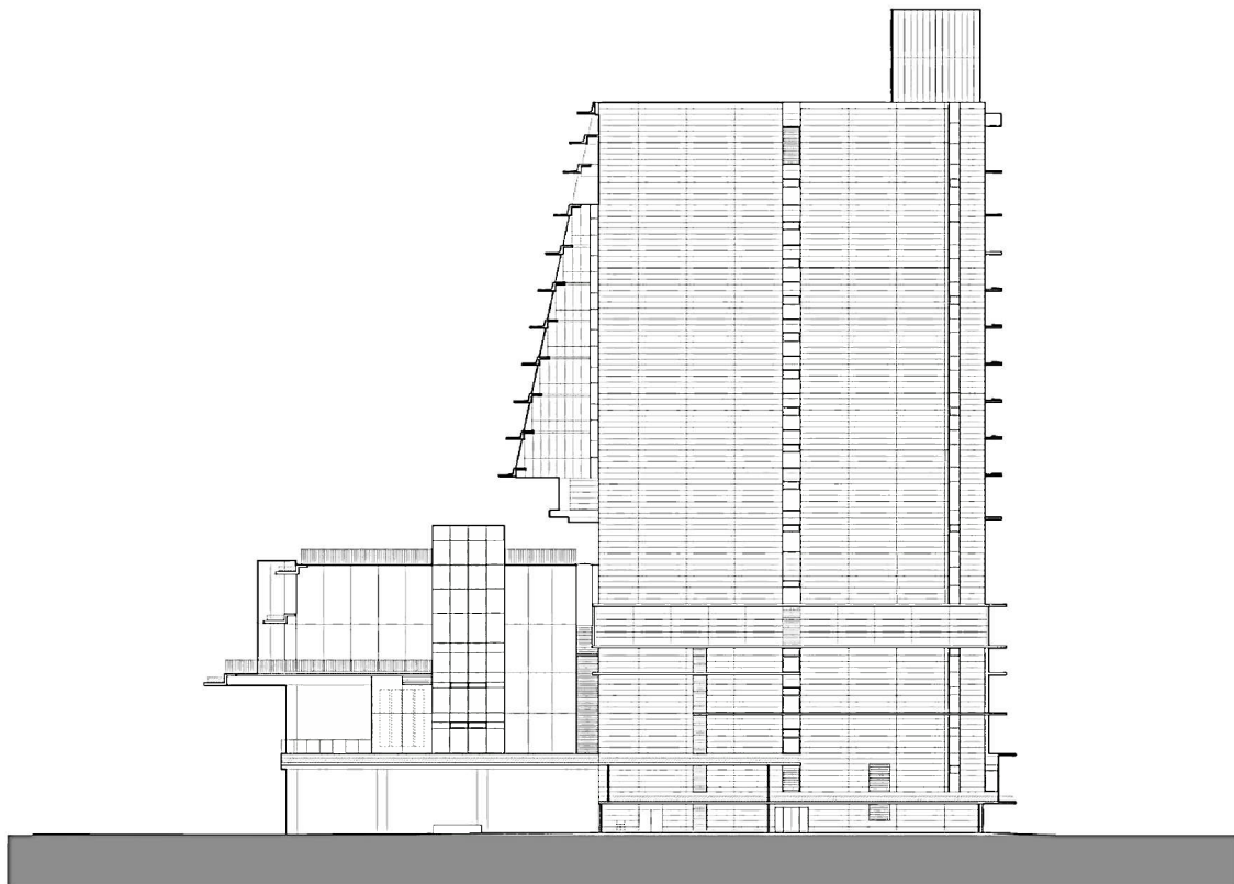
西立面图
