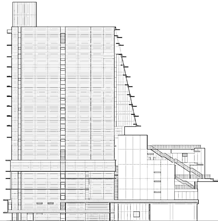
北立面图
