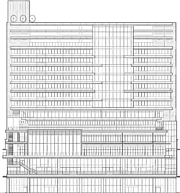
北立面图
