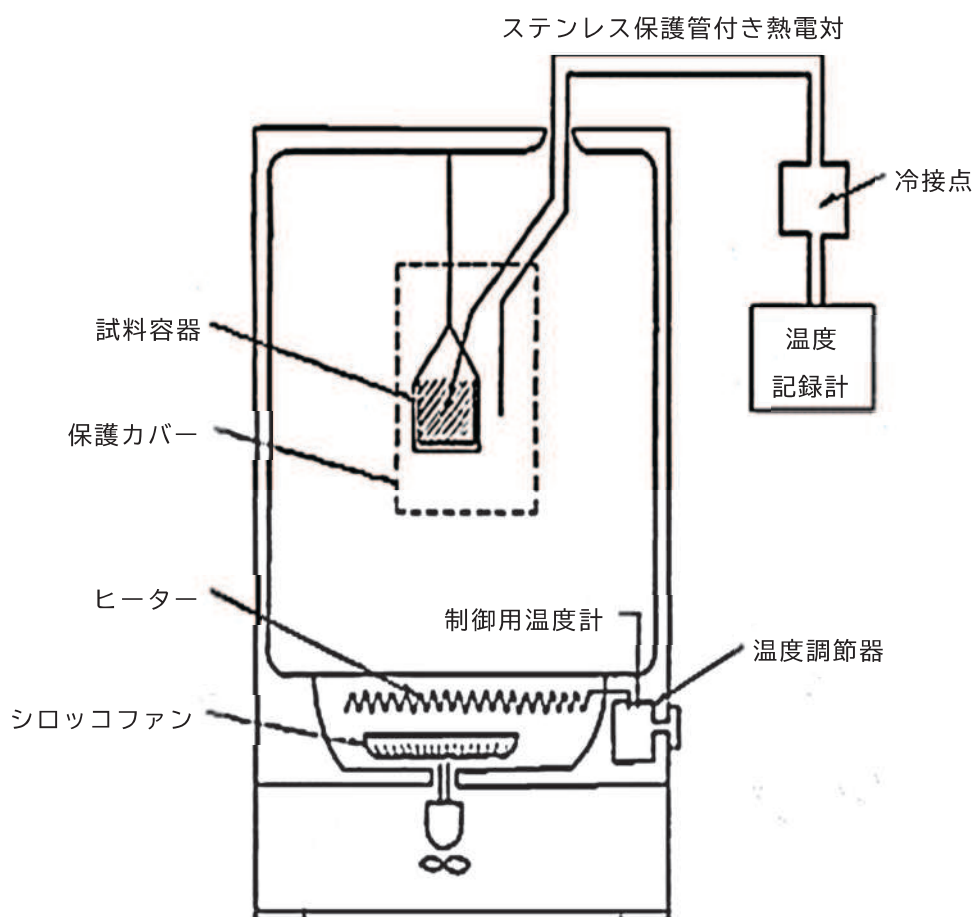
【第 10-1 図 自己発熱性物質の試験装置】
