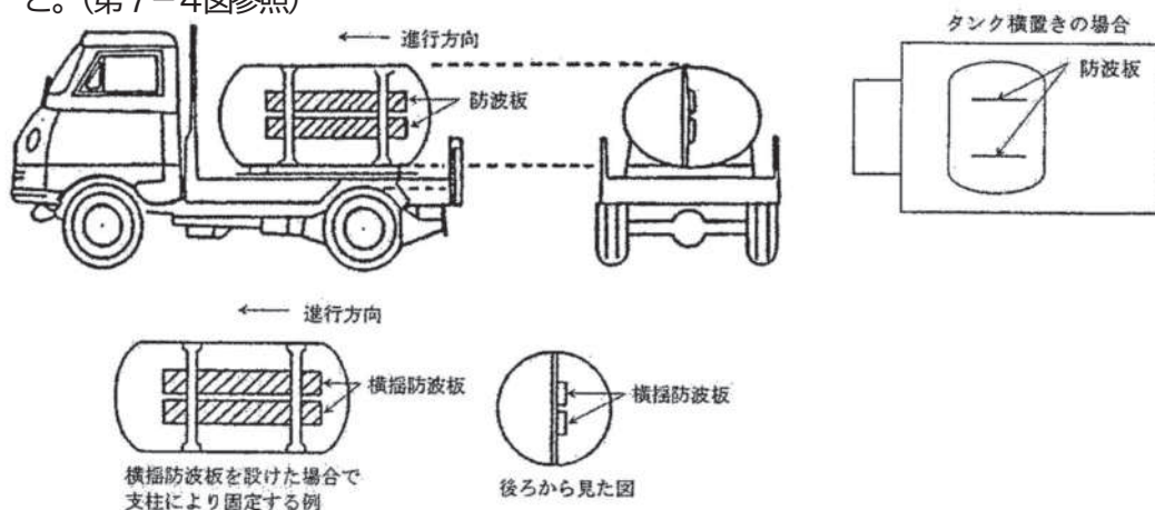
第7-4図 防波板の設置例
