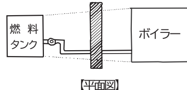
第5-5図 防火上有効な遮へいの例
