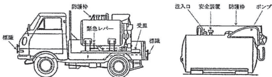
第7-7図 防護枠の例
