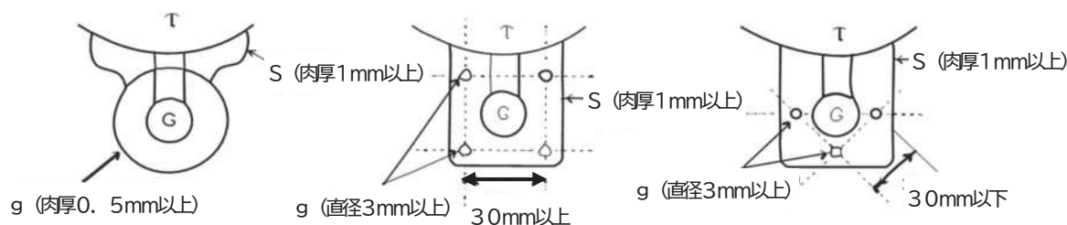
第5-4図 ガラスゲージの例
