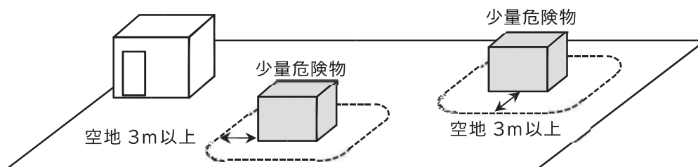
第1-16図 保有空地例により複数設置する場合
