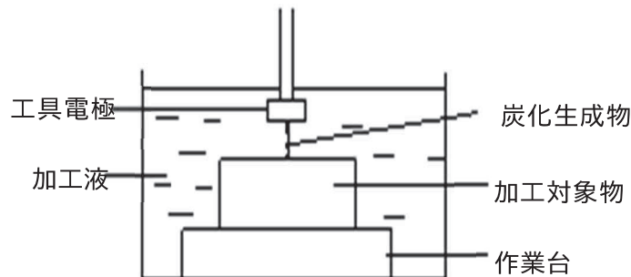
【第6-4図 炭化生成物発生例】
