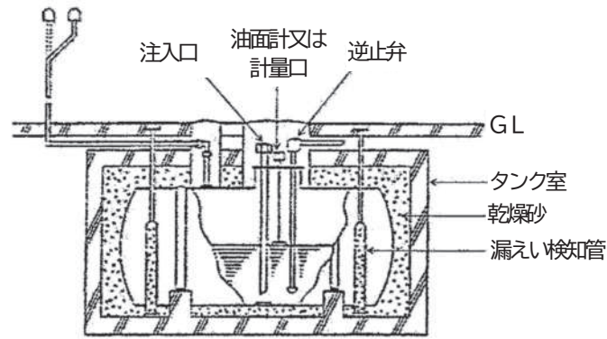
第6-1図 タンク室に設置する例
