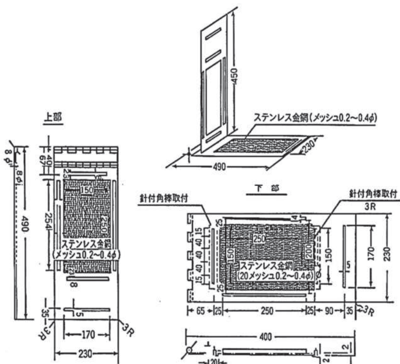
【第8－2図 試験体支持枠】単位:mm
