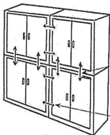
【第 1 - 2 図 薬品戸棚等固定方法の例】
