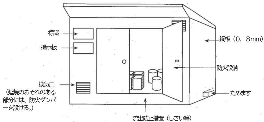
第4-9図 スチール製の貯蔵車により容器を貯蔵し、又は取り扱う場合の例
