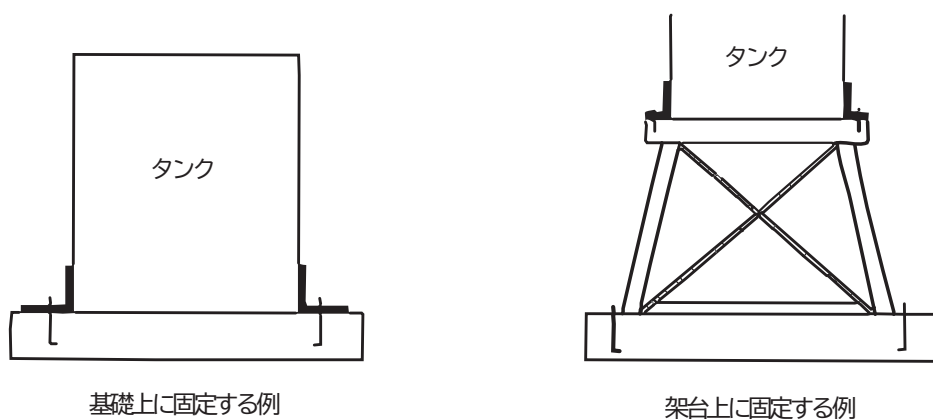
第5－2図 タンクの固定例
