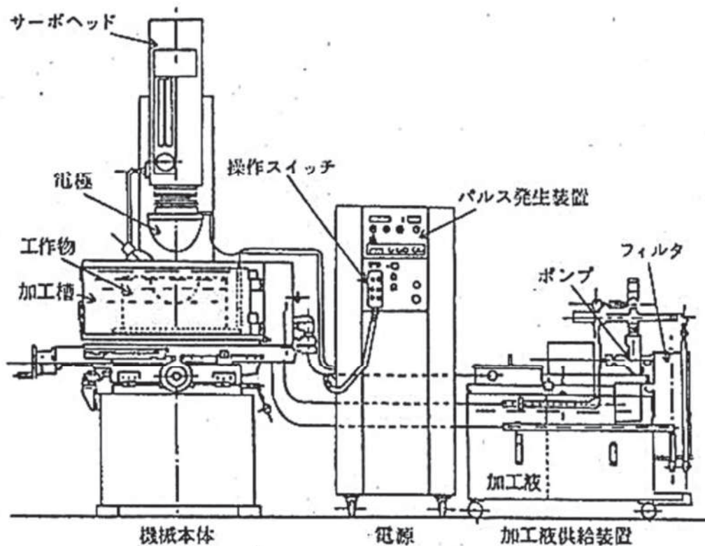
【第6－1図 放電加工機の構造図】
