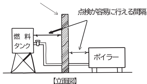
第5-5図 防火上有効な遮へいの例
