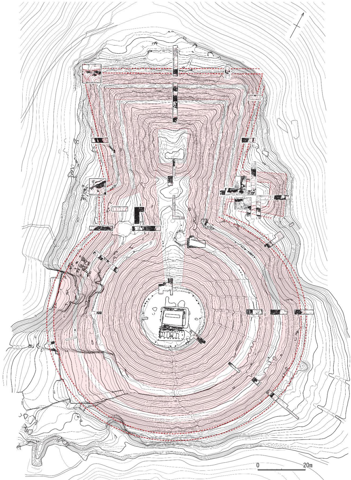
墳丘復元図
